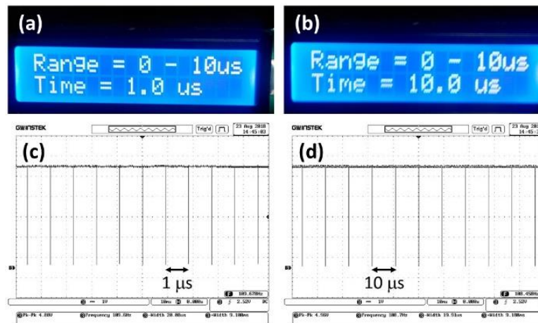
Gambar 3. Pulsa keluaran dari mikrokontroler rentang 0-10 \mu\text{s} : (a) dan (b) tampilan LCD nilai 1 dan 10 \mu\text{s} , (c) dan (d) bentuk pulsa di osiloskop nilai interval 1 dan 10 \mu\text{s}
