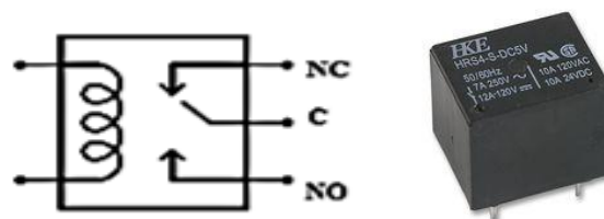
Gambar 4. Relai SPDT: rangkaian (kiri), fisik (kanan)
