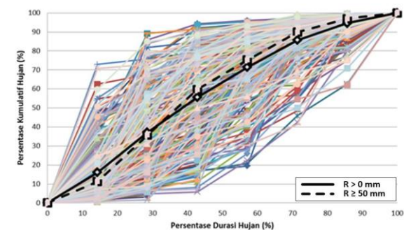
Gambar 10. Pola distribusi hujan rerata durasi 7 jam
