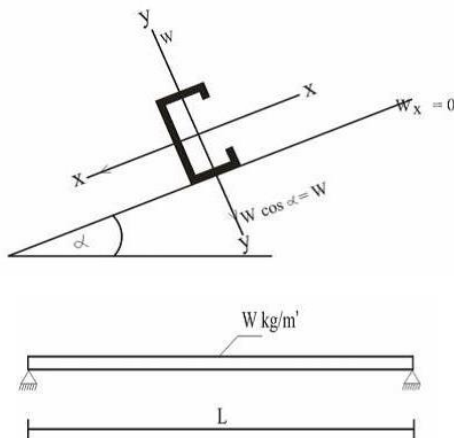
Gambar 5. Gaya yang bekerja pada beban angin
