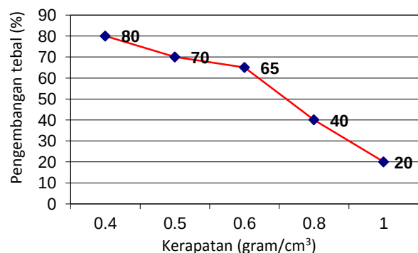
Gambar 9. Grafik penyerapan air
