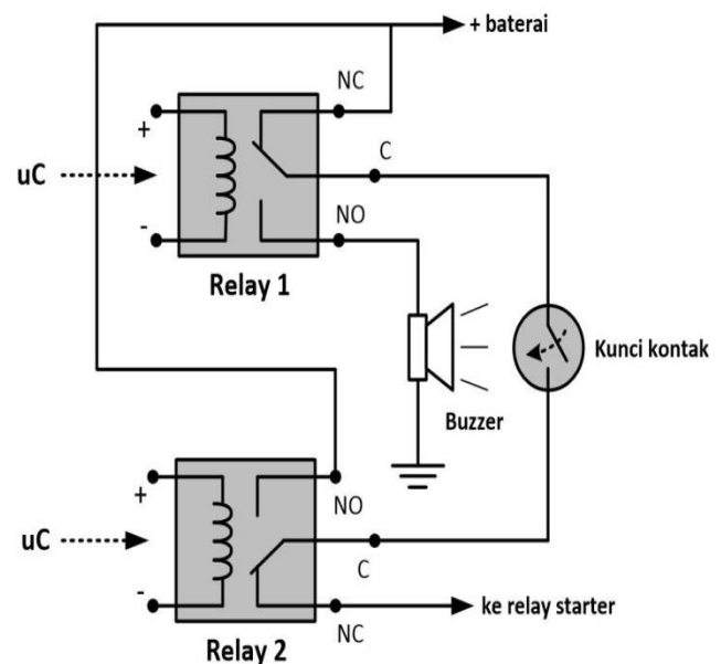
Gambar 7. Skema pensaklaran
