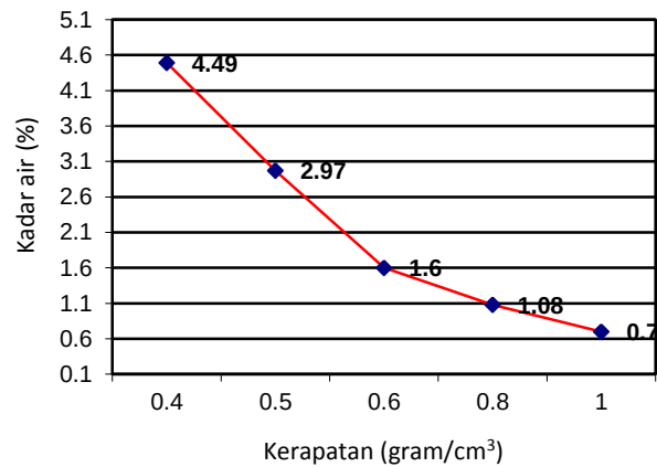
Gambar 6. Grafik kadar air
