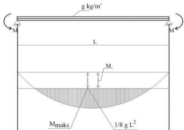
Gambar 3. Momen akibat beban mati
