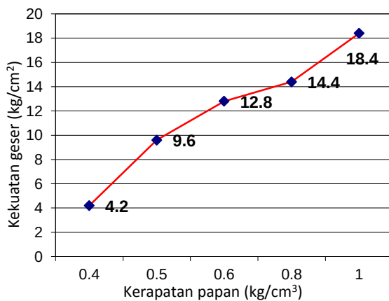
Gambar 12. Grafik kekuatan geser
