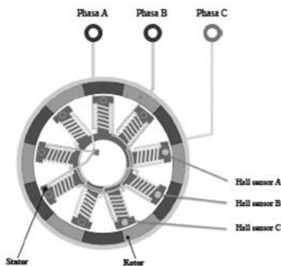
Gambar 2. Ilustrasi konstruksi MASTS dengan sensor hall
