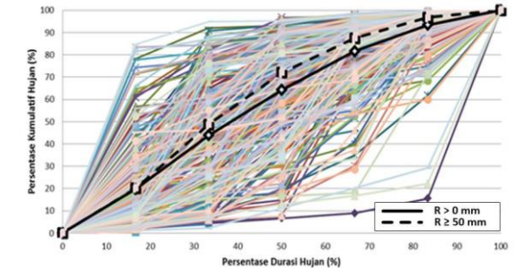
Gambar 9. Pola distribusi hujan rerata durasi 6 jam
