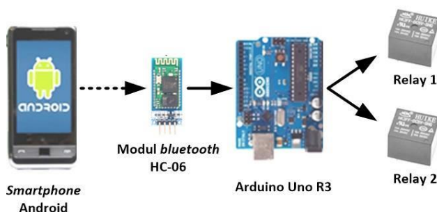
Gambar 6. Konfigurasi perangkat keras
