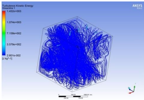
Gambar 4. Simulasi aliran varian 3
