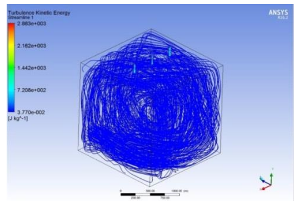
Gambar 6. Simulasi aliran varian 5
