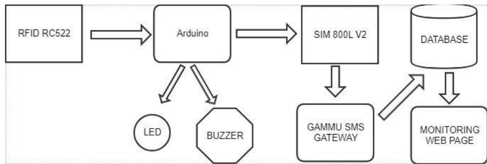
Gambar 1. Diagram blok sistem
