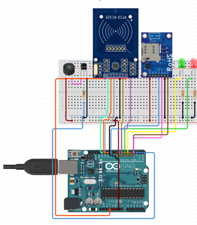
Gambar 2. Rancangan elektrik sistem
