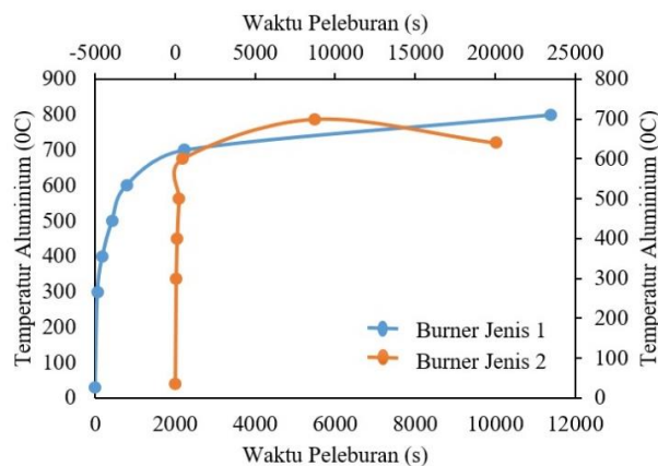
Gambar 6. Grafik distribusi temperatur dan waktu peleburan aluminium dengan letak burner di atas menggunakan burner jenis 1 dan burner jenis 2
