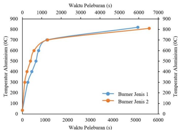
Gambar 5. Grafik distribusi temperatur dan waktu peleburan aluminium dengan letak burner di samping menggunakan burner jenis 1 dan burner jenis 2
