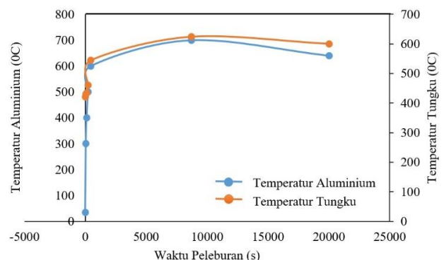
Gambar 9. Grafik perubahan temperatur aluminium, temperatur tungku, dan waktu peleburan dengan letak burner di atas serta burner jenis 2
