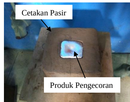
Gambar 3. Hasil penuangan cairan aluminium
