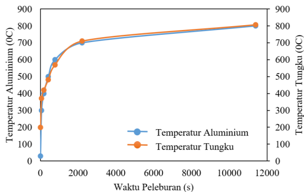
Gambar 8. Grafik perubahan temperatur aluminium, temperatur tungku dan waktu peleburan dengan letak burner di atas serta burner jenis 1.
