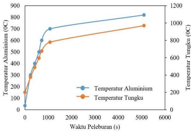
Gambar 7. Grafik perubahan temperatur aluminium, temperatur tungku dan waktu peleburan dengan letak burner di samping dan burner jenis 1
