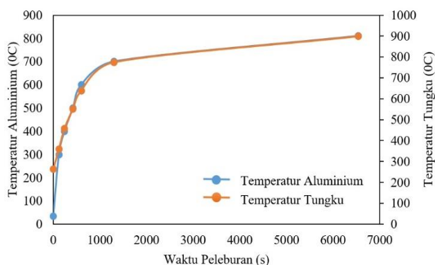
Gambar 10. Grafik perubahan temperatur aluminium, temperatur tungku, dan waktu peleburan dengan letak burner di samping dan burner jenis 2
