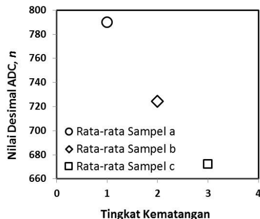
Gambar 9. Pengukuran nilai desimal konversi ADC terhadap tingkat kematangan Stroberi
