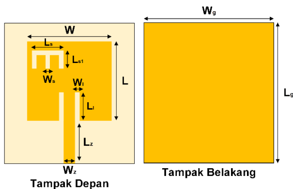
Gambar 2. Desain antena mikrostrip dengan penambahan slot M dan inset
