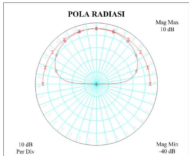
Gambar 10. Pola radiasi antenna mikrostrip dengan penambahan slot M dan inset
