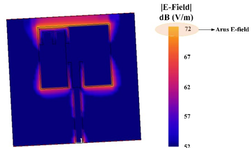
Gambar 9. Arus E-field antenna mikrostrip dengan penambahan slot M dan inset
