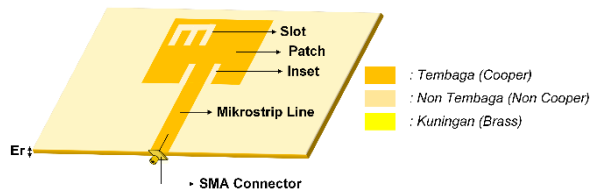
Gambar 3. Struktur antena mikrostrip dengan penambahan slot M dan inset
