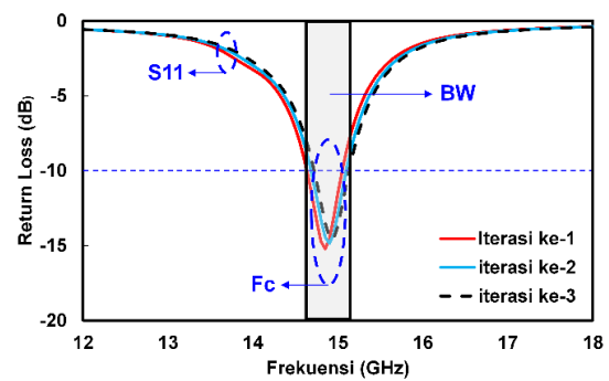
Gambar 6. Hasil simulasi return loss dari iterasi panjang slot ( L_s ) dan ( L_{s1} )
