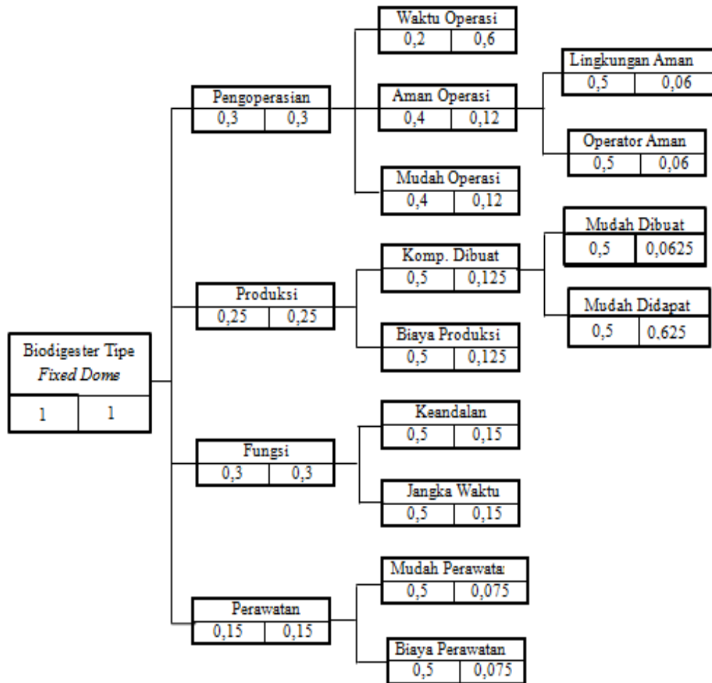
Gambar 10. Pohon keputusan
