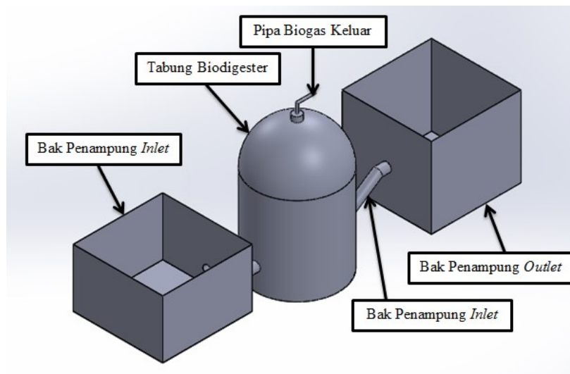
Gambar 11. Desain biodigester tipe fixed dome
