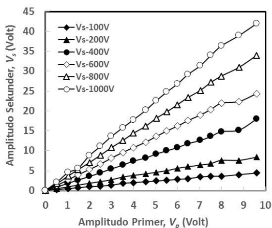
Gambar 7. Pengaruh amplitudo primer terhadap amplitudo sekunder untuk tiap terminal sekunder
