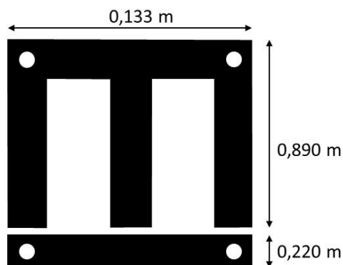
Gambar 3. Inti besi transformator
